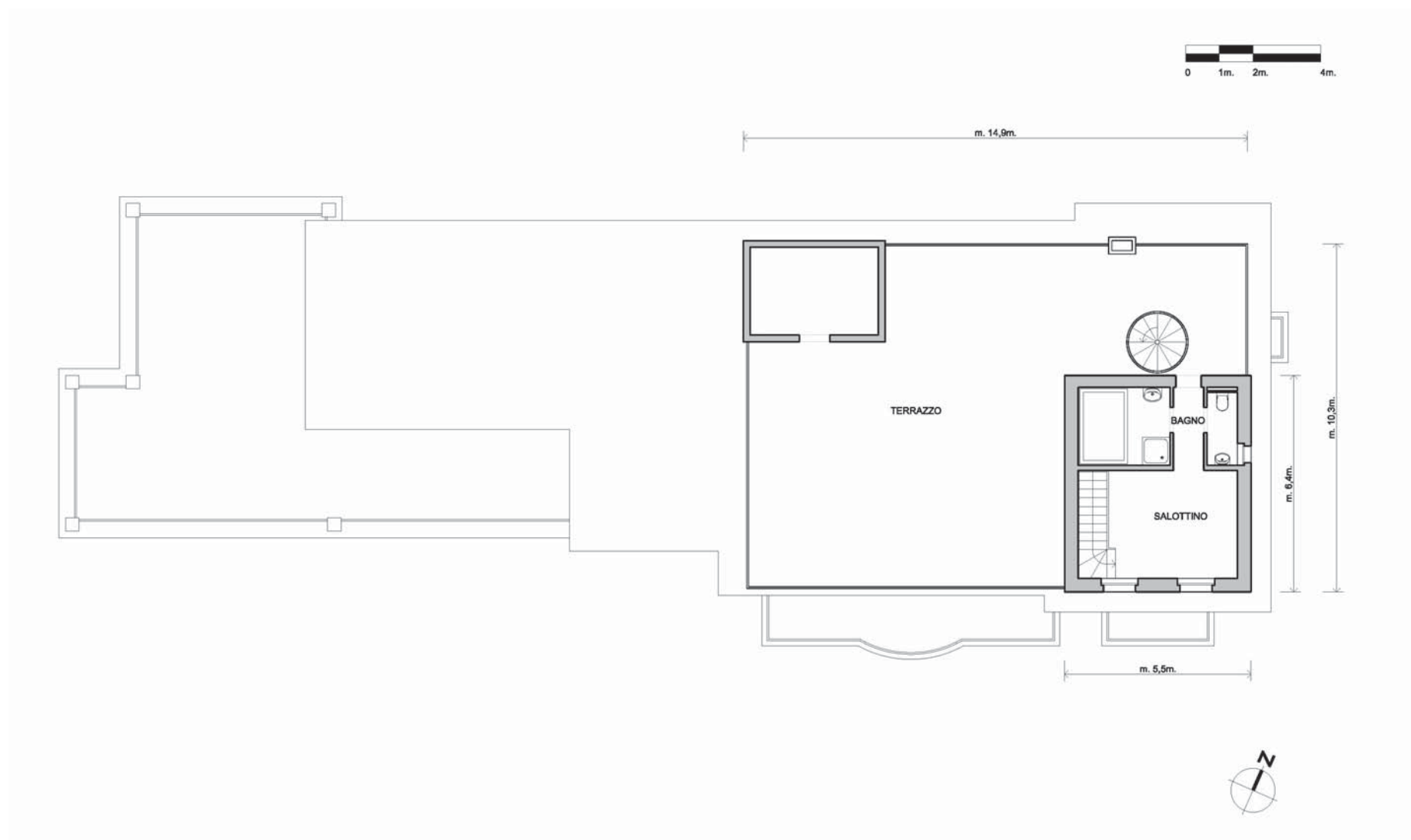
6°PIANO, STATO ATTUALE - 6° FLOOR, PRESENT SITUATION
