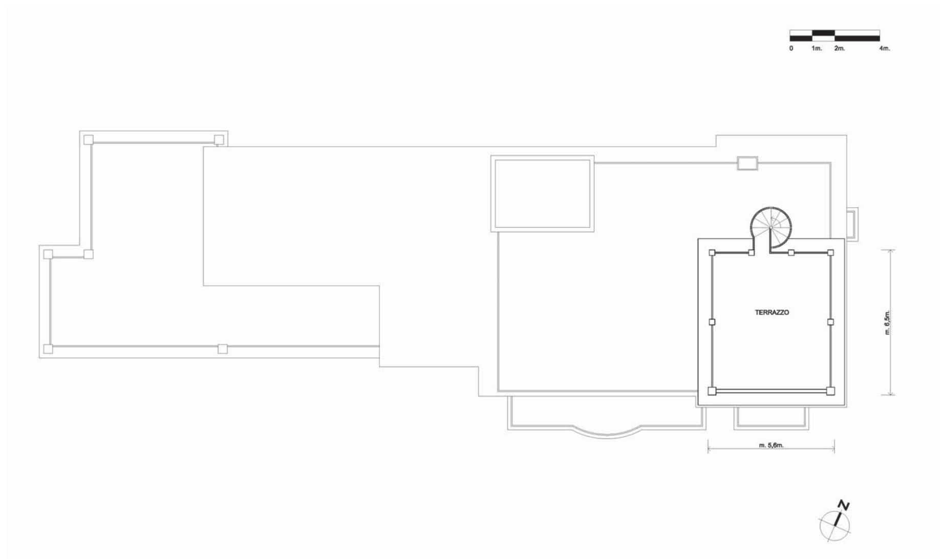
7° PIANO, NUOVO PROGETTO - 7° FLOOR PLAN, NEW PROJECT
