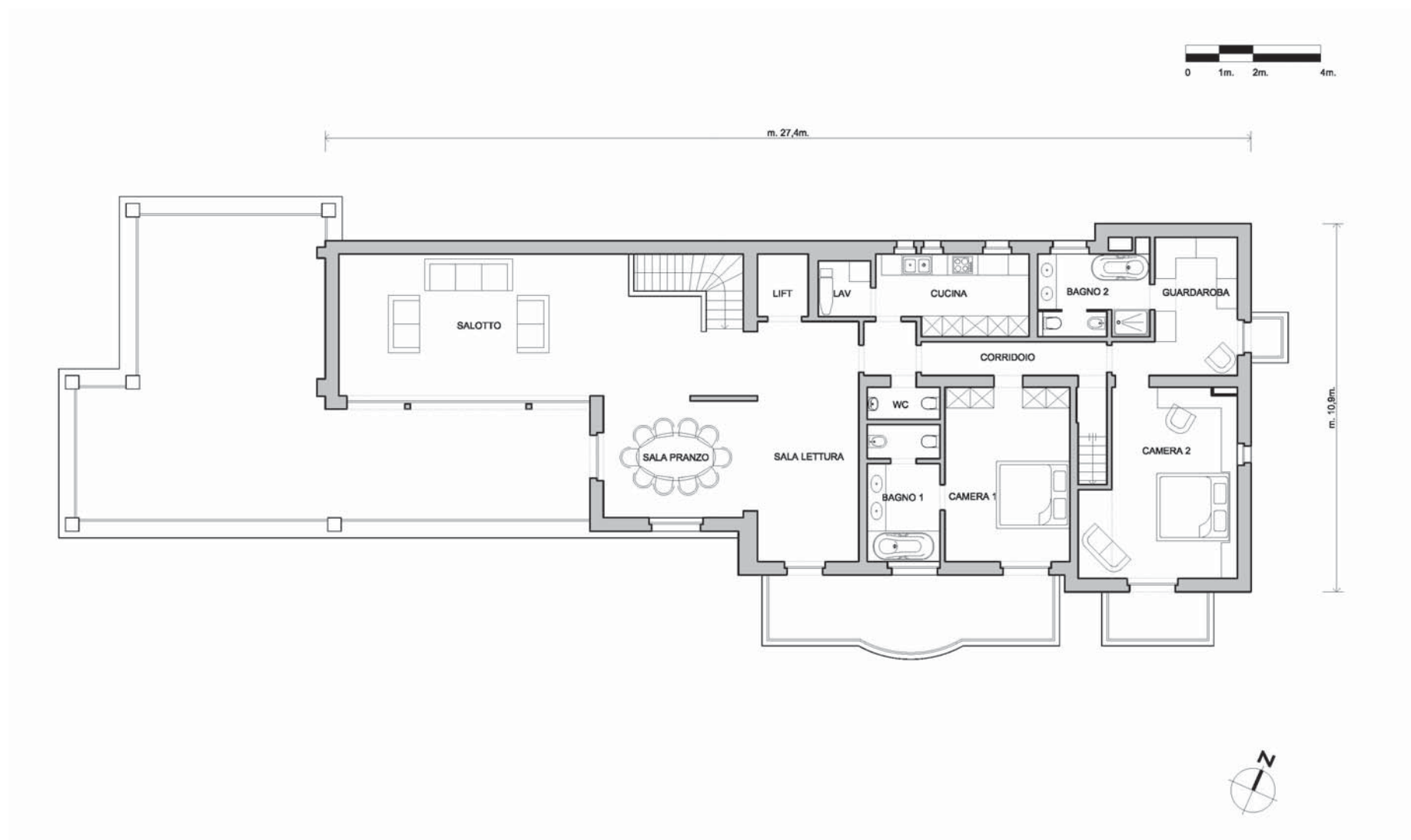
5° PIANO, NUOVO PROGETTO OPZ. 1 - 5° FLOOR PLAN, NEW PROJECT OPT. 1
