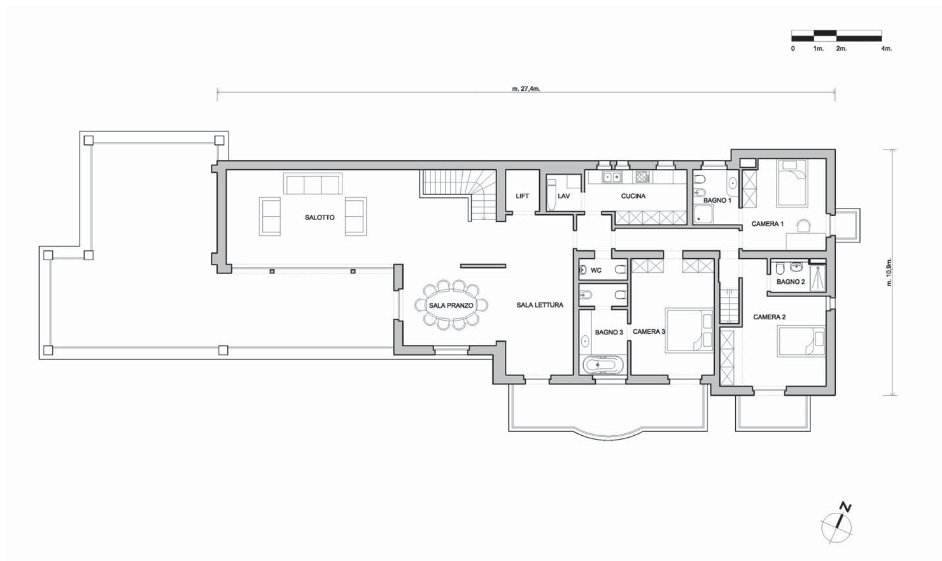
5° PIANO, NUOVO PROGETTO OPZ. 2 - 5° FLOOR PLAN, NEW PROJECT OPT. 2
