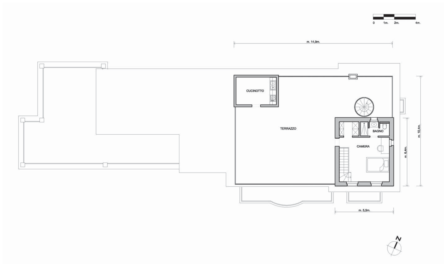
6° PIANO, NUOVO PROGETTO - 6° FLOOR PLAN, NEW PROJECT
