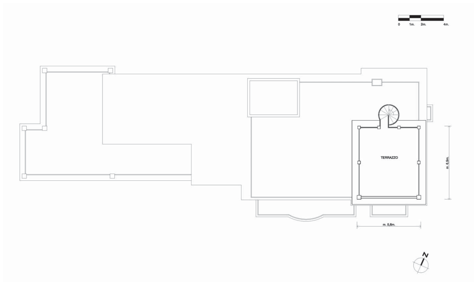
7° PIANO, STATO ATTUALE - 7° FLOOR, PRESENT SITUATION
